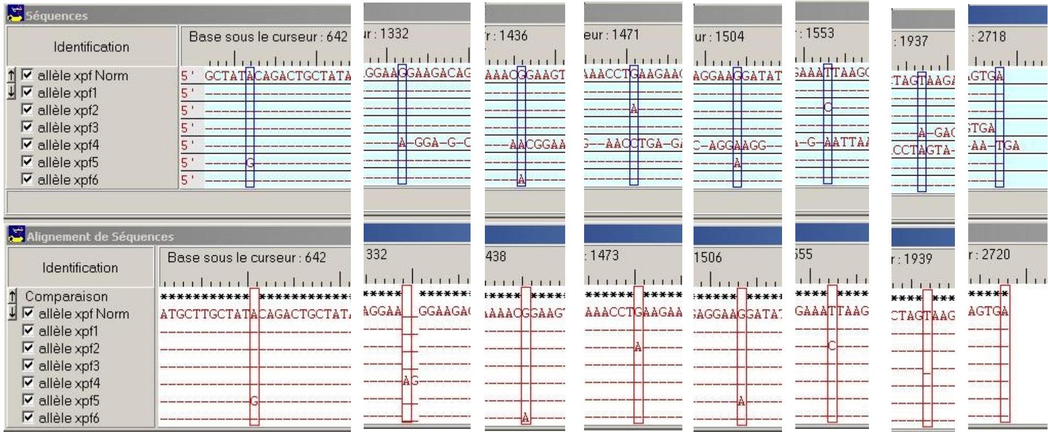
Comparaison de différentes séquences ADN du gène xpf (logiciel GénieGen)
